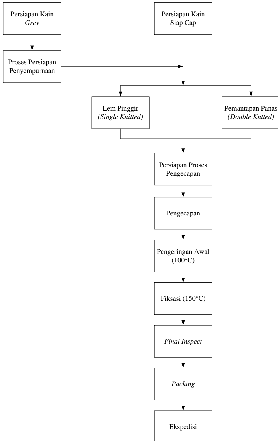
Gambar I- 1 Alur Proses Produksi Kain
