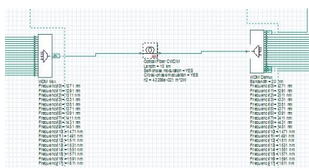
Gambar 7, Blok Jaringan
