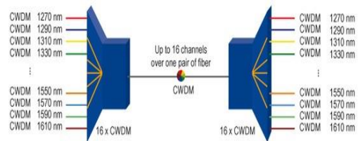
Gambar 2 Pajang Gelombang CWDM [7]
