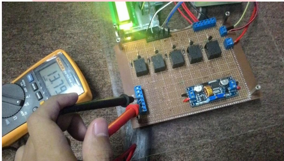
Gambar 4.3 Pengujian Relay
