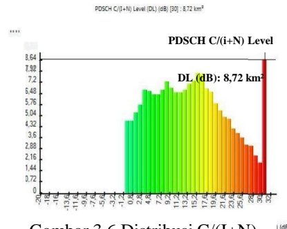
Gambar 3.6 Distribusi C/(I+N) Bandung - Cikampek
