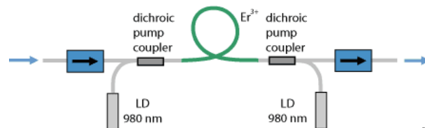
Gambar 4 Skema penguatan optik menggunakan EDFA [7]
