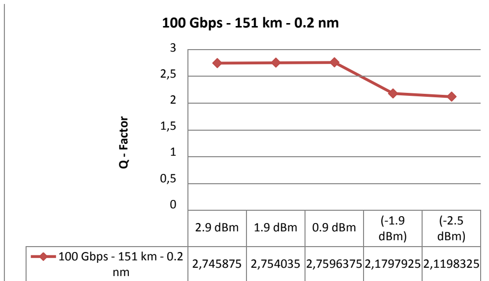
Gambar 14 Pengaruh daya transmitter pada bitrate 100 Gbps, jarak 151 km, dan spasi kanal 0.2 nm
