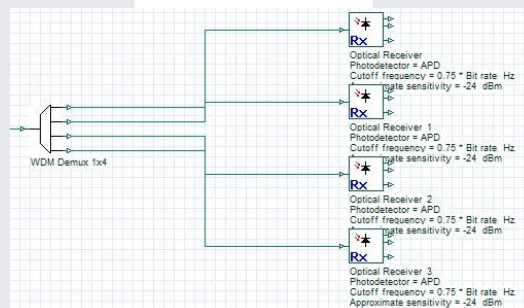
Gambar 9 Blok penerima
