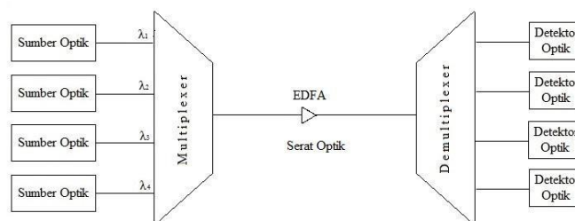
Gambar 5 Diagram blok sistem
