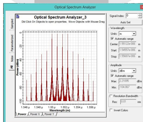
Gambar 8 Spektrum sinyal dengan indeks bias non linear
