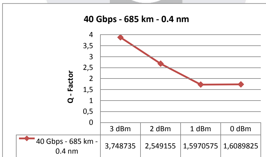
Gambar 13 Pengaruh daya transmitter pada bitrate 40 Gbps, jarak 685 km, dan spasi kanal 0.4 nm
