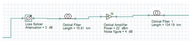
Gambar 10 Blok transmisi
