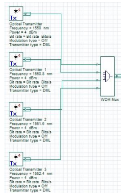
Gambar 6 Blok Pengirim
