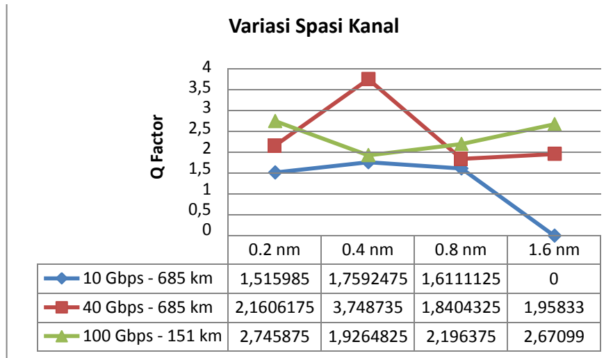
Gambar 11 Pengaruh spasi kanal pada bitrate 10, 40, dan 100 Gbps
