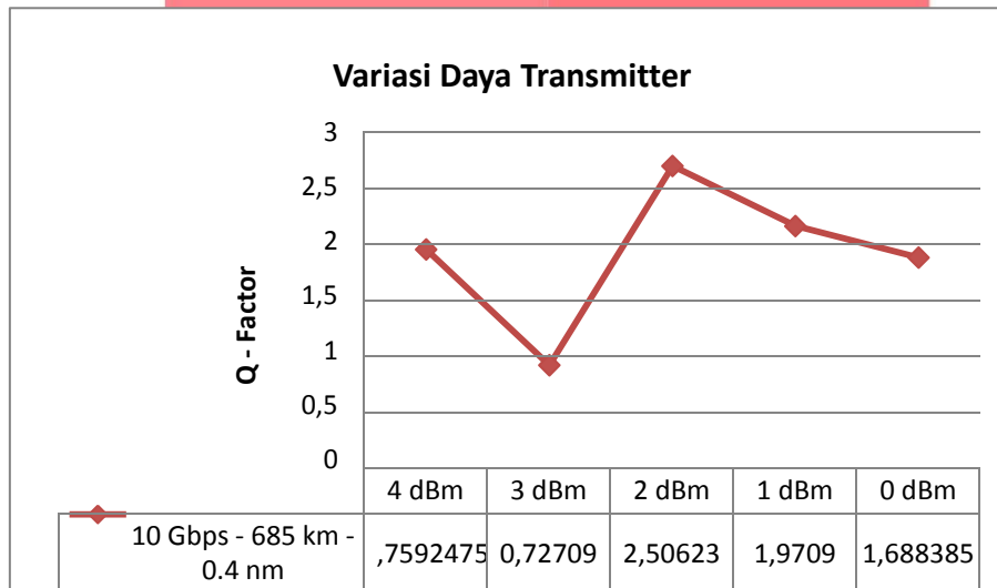
Gambar 12 Pengaruh daya transmitter pada bitrate 10 Gbps, jarak 685 km, dan spasi kanal 0.4 nm
