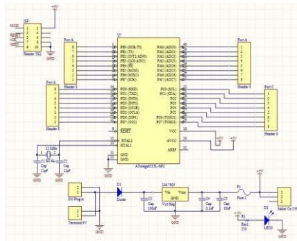
Gambar 3.2 Sismin Mikrokotroller
