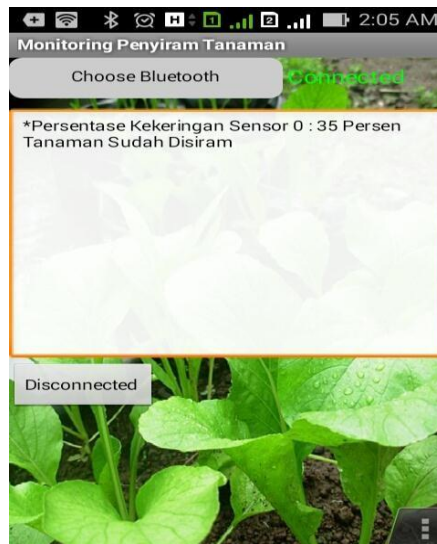
Gambar 3.6 Tampilan Aplikasi
