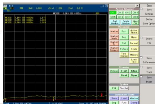
Gambar 6 (a) Grafik VSWR Pada Frekuensi ( 3.1 – 10.6) GHz di Free Space , (b) VSWR Antena pada Frekuensi (3.1-10.6) GHz saat Free Space
