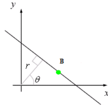
Gambar 2.2 Citra sebuah garis dalam Kartesian dengan satu titik uji [3]
