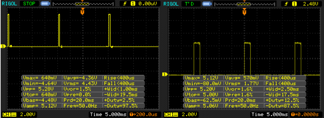
Gambar 4.3. 1 PWM 2,5%
