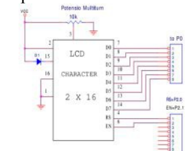
Gambar 2. 14 Skematik Rangkaian Interface LCD
