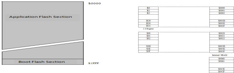
Gambar 2.8 Peta Memori ATmega16 Gambar 2.9 Konfigurasi Memori Data ATmega16
