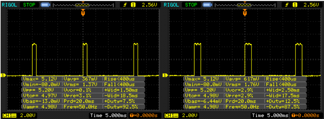
Gambar 4.2. 1 PWM 7,5
