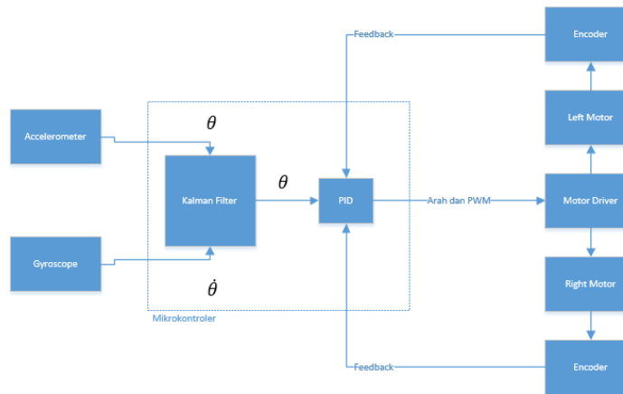
Gambar 10. Blok diagram sistem
