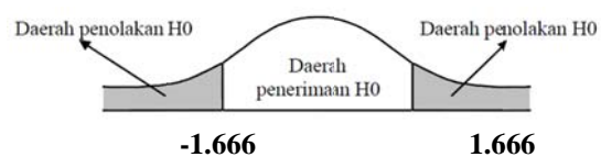
Kurva Uji Parsial Variabel Tempat
