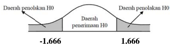
Kurva Uji Parsial Variabel Produk
