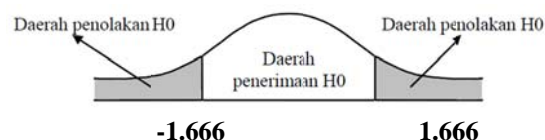
Kurva Uji Parsial Variabel Harga
