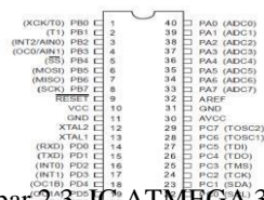
Gambar 2.3 IC ATMEGA 32
