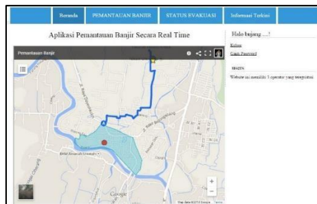
Gambar 4.6 Antarmuka Aplikasi
