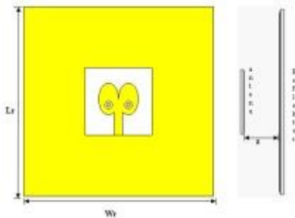
Gambar : Antenna dual elip dengan slot dan reflector Sebelum ditetapkan untuk menggunakan reflektor dianalisis terlebih dahulu perbandingan parameter VSWR, range frekuensi dan Gain antara Antenna yang belum dipasangkan reflektor dan antenna yang sudah dipasangkan reflektor.
