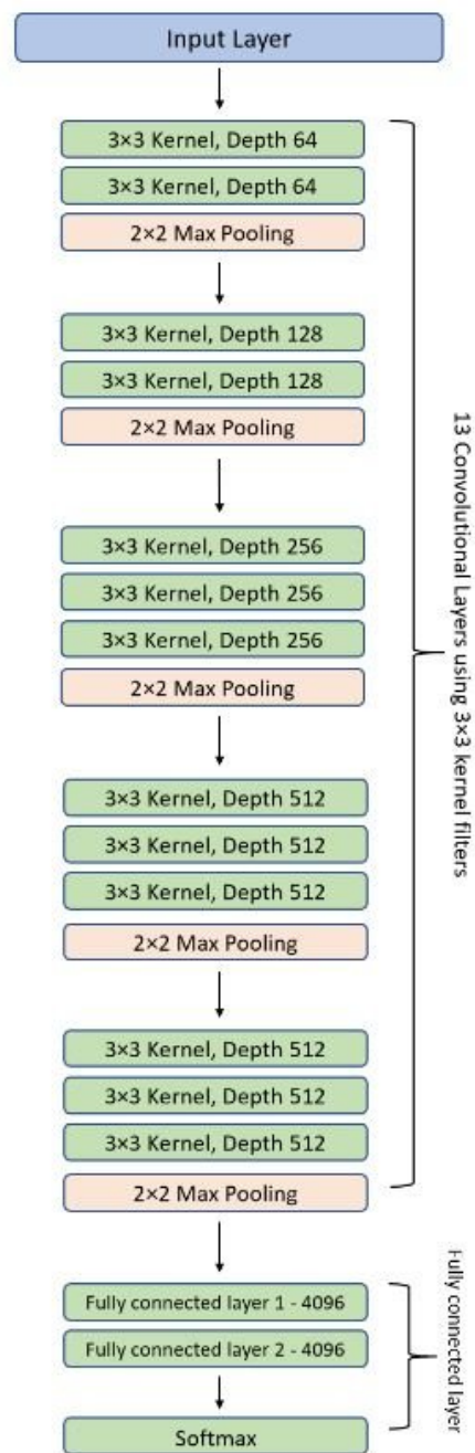
Gambar 1. Arsitektur VGG-16 [15]
