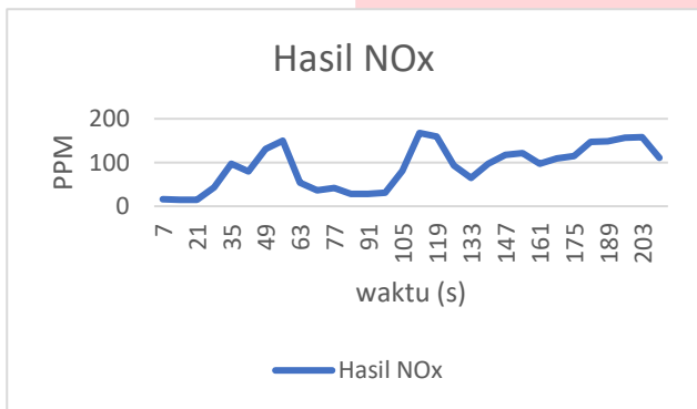
GAMBAR 4.3 Grafik Pengujian NOx
