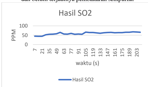
GAMBAR 4.4 Grafik Pengujian SO2
