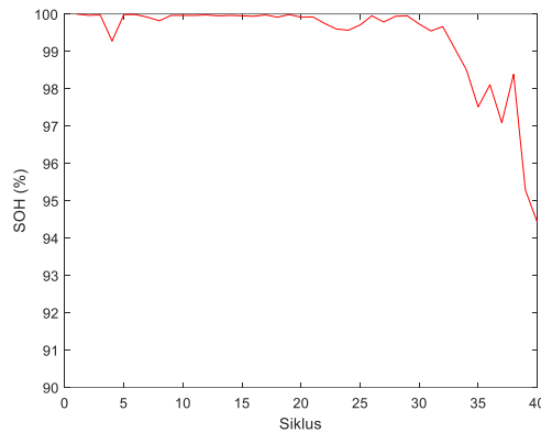
Gambar 4.4 Grafik SOH
