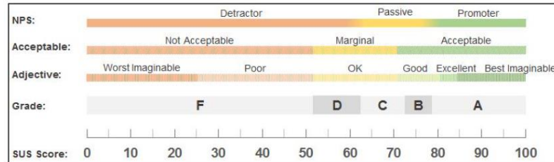
Gambar 3. SUS Card
