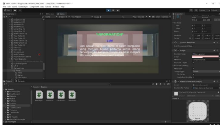
Gambar 13 Tampilan UI world space tampak belakang setelah ditambahkan script
