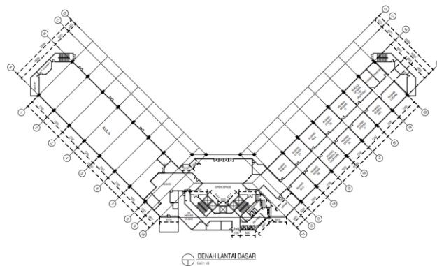
Gambar 3 Sketsa Denah Gedung Kampus Institut Teknologi Telkom Surabaya
