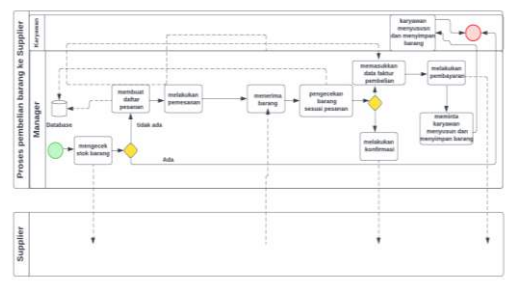
GAMBAR 3 BPMN
