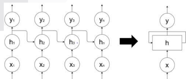
GAMBAR 2.3 ARSITEKTUR SEDERHANA RNN
