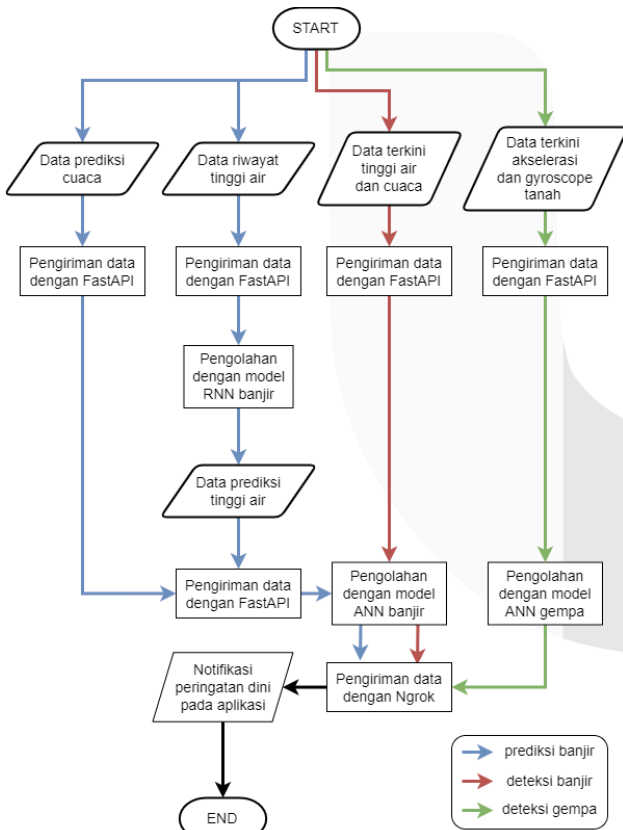
GAMBAR 4.24 DIAGRAM ALIR KERJA APLIKASI
