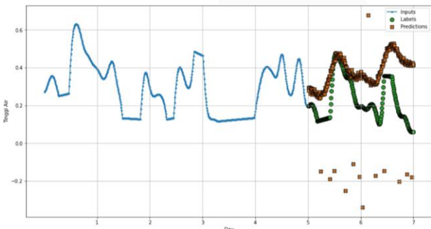
GAMBAR 4.18 GRAFIK HASIL PREDIKSI MODEL LSTM DENGAN DATA SMOOTHING
