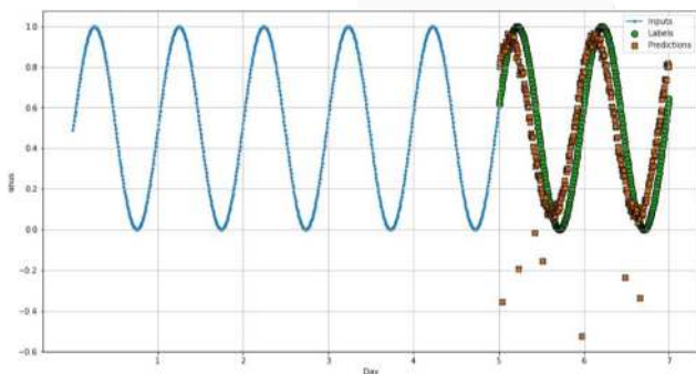
GAMBAR 4.15 GRAFIK HASIL PREDIKSI MODEL RNN DENGAN DATA SINUS
