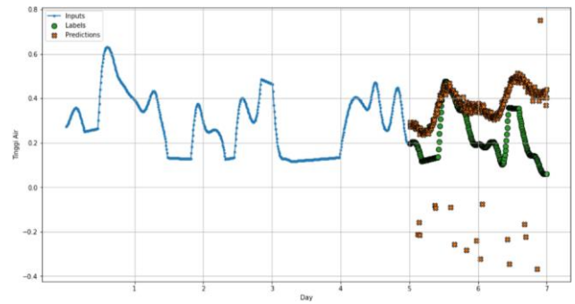
GAMBAR 4.19 GRAFIK HASIL PREDIKSI MODEL LSTM DALAM 4 KALI PERCOBAAN
