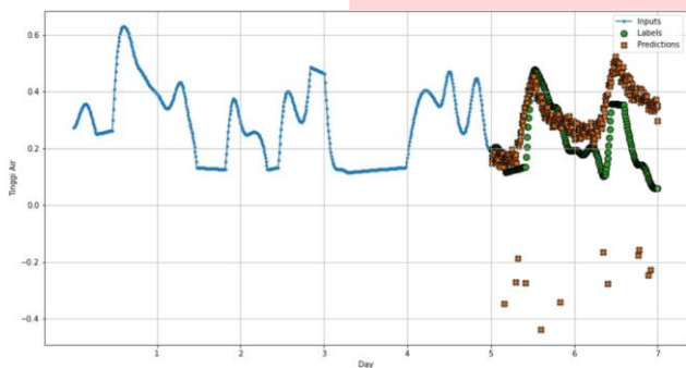
GAMBAR 4.13 GRAFIK HASIL PREDIKSI MODEL RNN DENGAN DATA SMOOTHING
