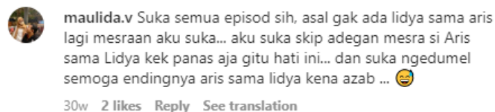
Gambar 1.4 Komentar Netizen
