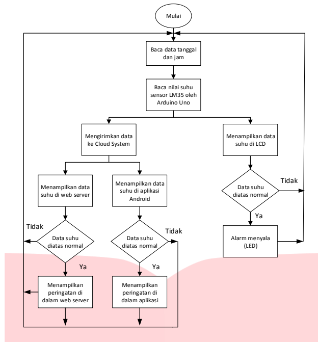
Gambar 5 Alur Kerja Sistem Mikrokontroller
