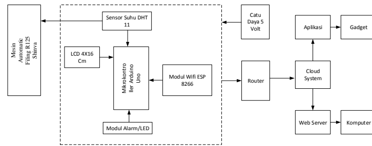
Gambar 3 Prinsip Kerja Sistem
