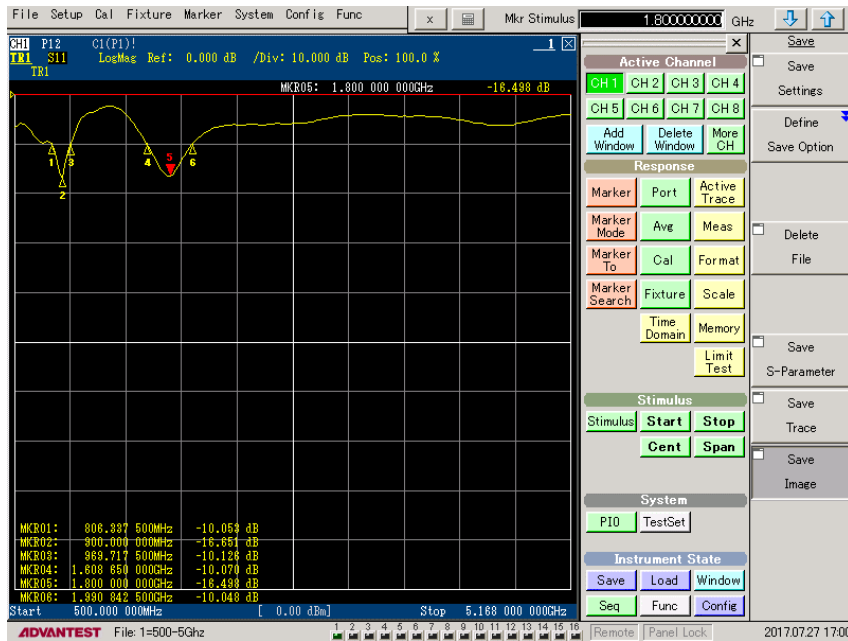
Gambar 4.2 Return Loss dan Bandwidth
