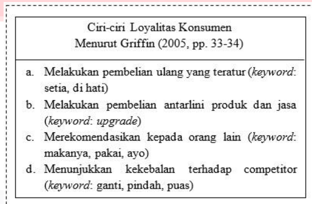
Gambar 2.2 Kerangka Pemikiran
