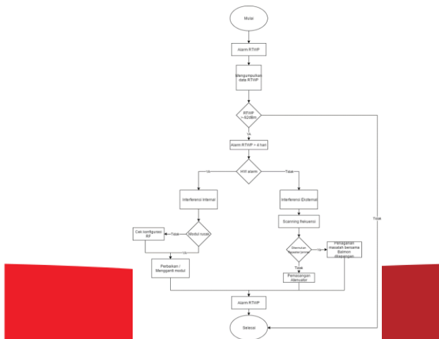
Gambar 3.1.1 Diagram alur penanganan interferensi
