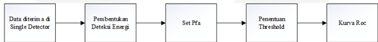
Gambar 6 Tahap-tahap Penentuan Threshold dan Kurva ROC menggunakan Deteksi Energi
