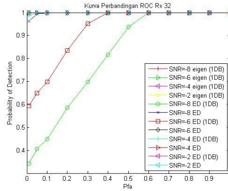
Gambar 16 Hasil Perbandingan Kurva ROC nr 32
