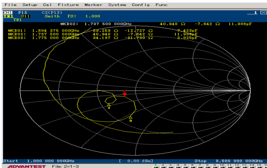
Gambar 4. 4 Hasil Pengukuran Impedansi
