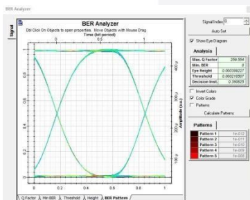
Gambar 11 Hasil optimasi link upstream pada Optisystem
