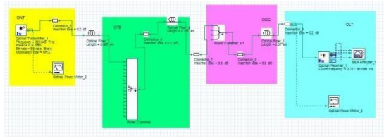
Gambar 10 Optimasi link upstream pada Optisystem
