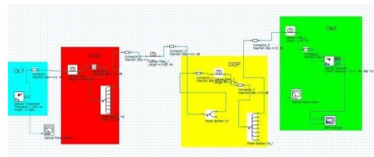
Gambar 3. Link downstream pada Optisystem
