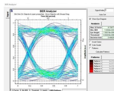
Gambar 9. BER analyzer Optisistem pada link downstream optimalisasi
