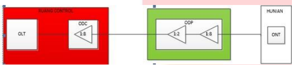
Gambar 2. Konfigurasi Umum
