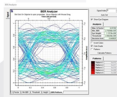
Gambar 4. BER Analyzer Optisystem pada link downstream
