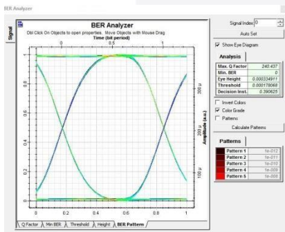
Gambar 7. BER Analyzer Optisystem pada link upstream
