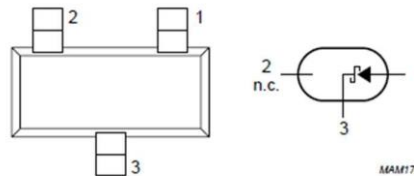
Gambar 1 Struktur BAT17 [7]
