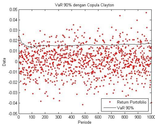
Figure 8: Grafik Nilai VaR Copula Clayton dengan tingkat kepercayaan 90%
