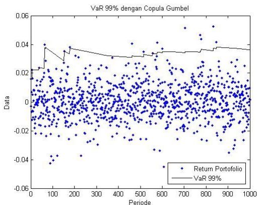
Figure 13: Grafik Nilai VaR Copula Gumbel dengan tingkat kepercayaan 99 %
