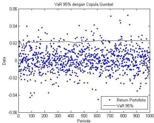
Figure 11: Grafik Nilai VaR Copula Gumbel dengan tingkat kepercayaan 95%
