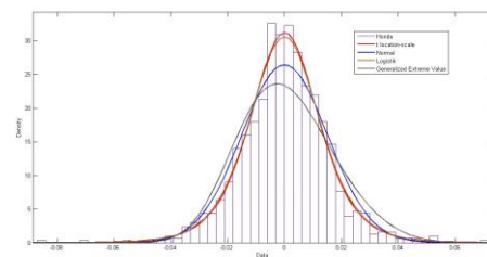
Figure 4: Uji kecocokan distribusi dengan histogram data return Honda
