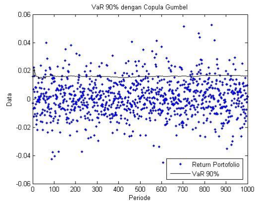
Figure 9: Grafik Nilai VaR Copula Gumbel tingkat kepercayaan 90%
