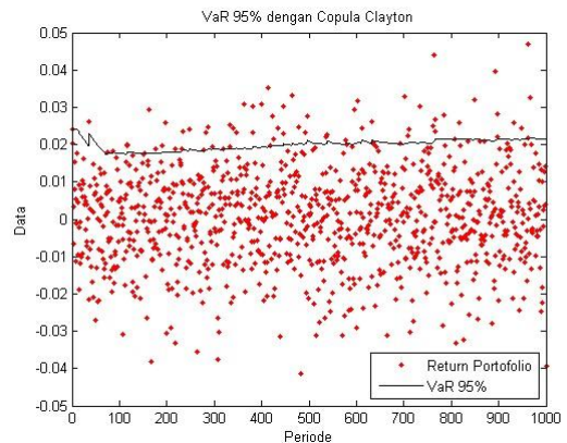
Figure 10: Grafik Nilai VaR Copula Clayton dengan tingkat kepercayaan 95%
