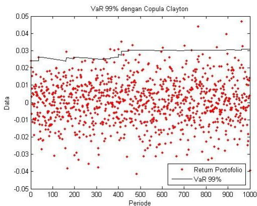
Figure 12: Grafik Nilai VaR Copula Clayton dengan tingkat kepercayaan 99 %
