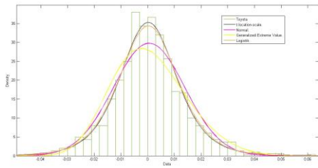
Figure 5: Uji kecocokan distribusi dengan histogram data return Toyota
