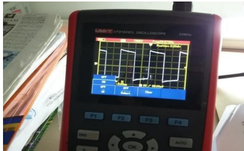
Gambar 7 Gelombang Output LM339 untuk Tegangan
