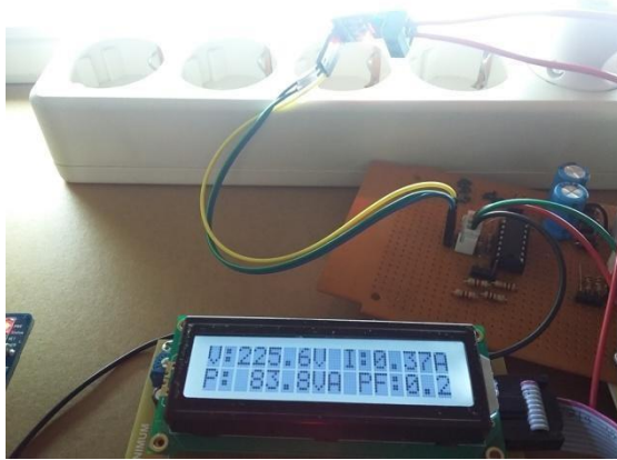
Gambar 12 Tampilan LCD dengan beban lampu TL 18w
