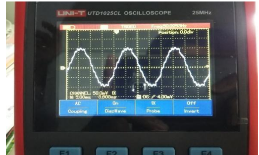
Gambar 6 Sinyal Keluaran Sensor Tegangan
