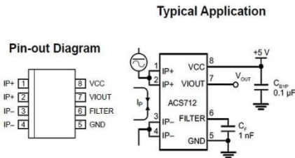
Gambar 4 ACS 712
