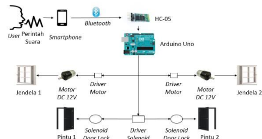
Gambar 3-1 Rancangan Sistem
