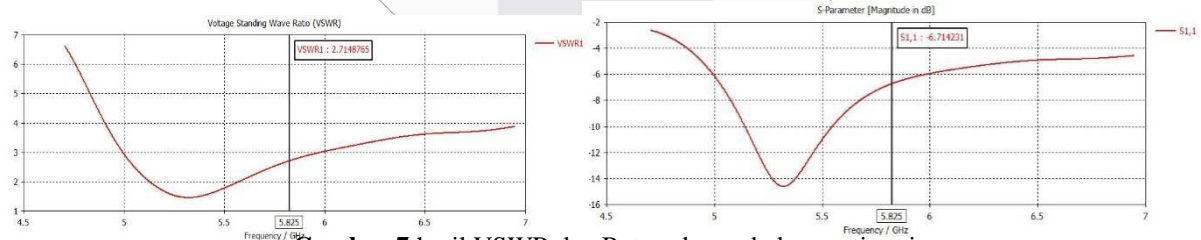
Gambar 7 hasil VSWR dan Return loss sebelum optimasi
