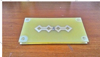
Gambar 8 hasil realisasi Antena
