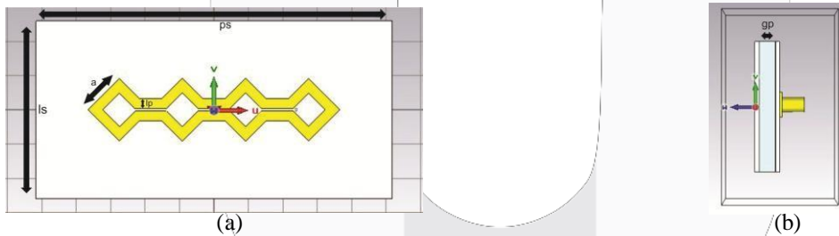
Gambar 6 simulasi antena (a).tampak depan (b) tampak samping
