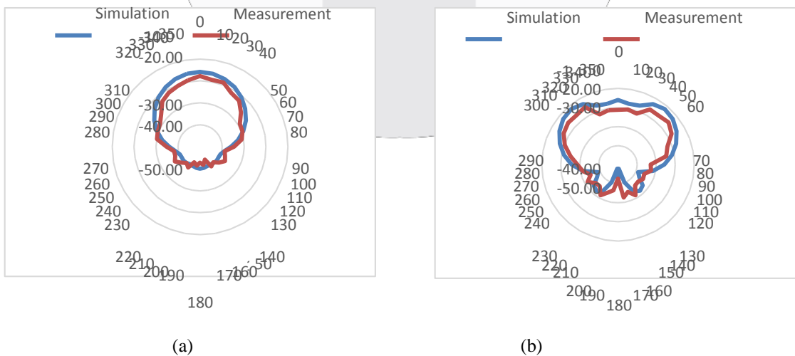
Gambar 12 Pola Radiasi (a)elevasi (b) azimuth
