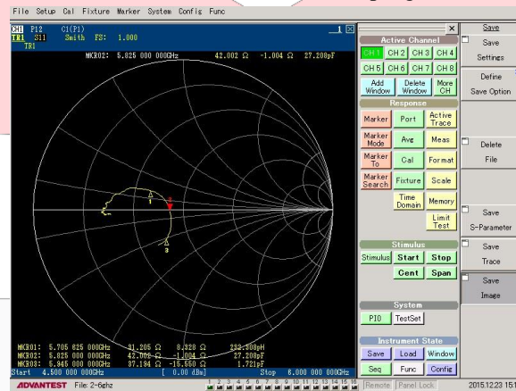
Gambar 11 Hasil pengukuran impedansi
