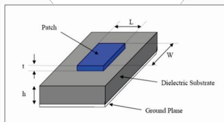
Gambar 1 Susunan Elemen Antena Mikrostrip [7]
