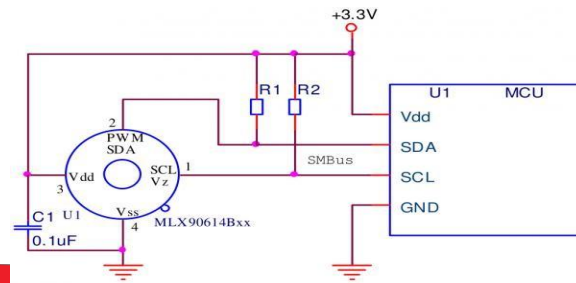
Gambar 2.3 Konektor MLX90614 SMBus
