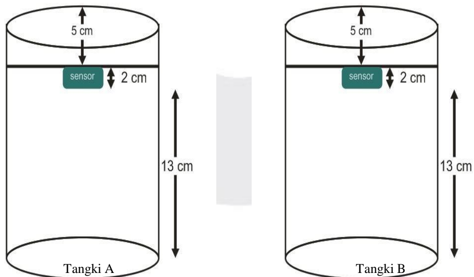
Gambar 2.3 Percontohan tangki
