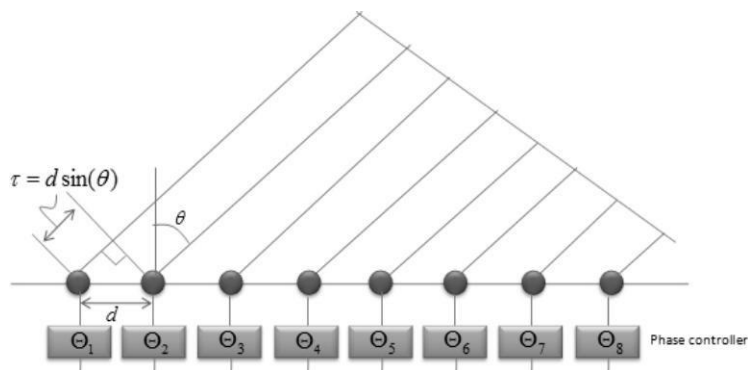
Gambar 1 Konsep beamforming
