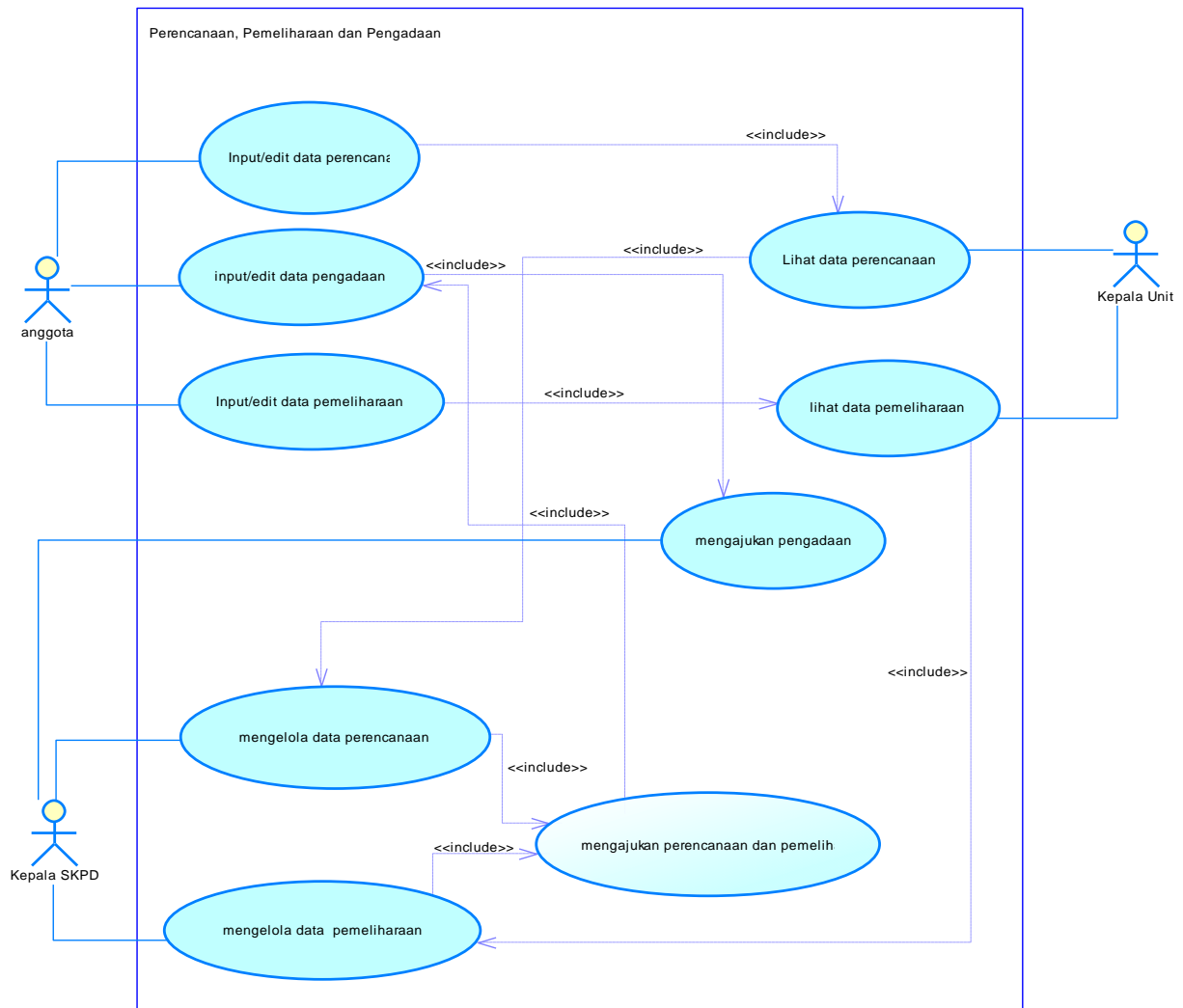
Gambar 3. Use Case Pengadaan, Pemeliharaan dan Pengadaan
