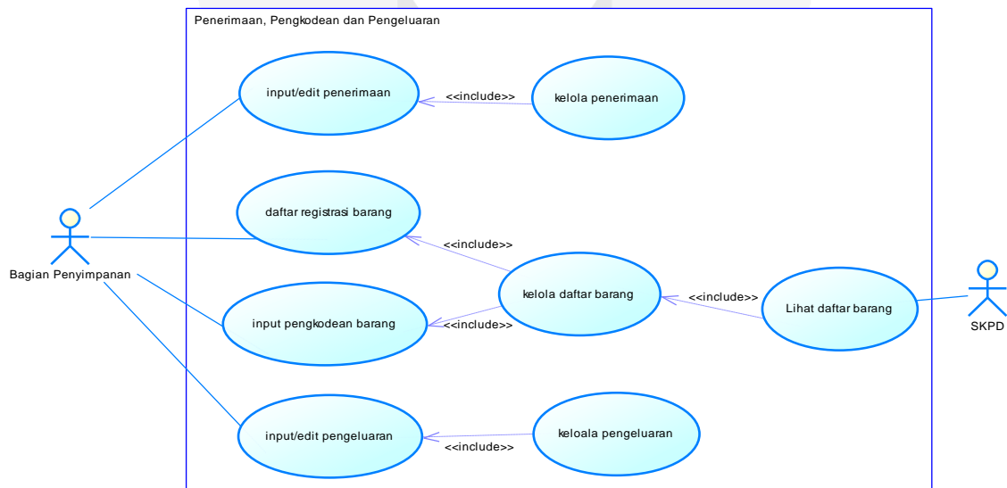
Gambar 4. Use Case Penerimaan, Pengkodean dan Pengeluaran
