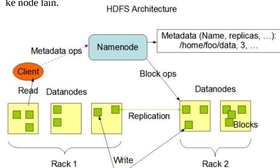
Gambar 1 Arsitektur HDFS
