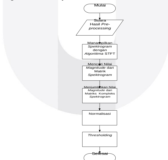
Gambar 3.4 Diagram Alir Proses Ekstraksi Ciri
