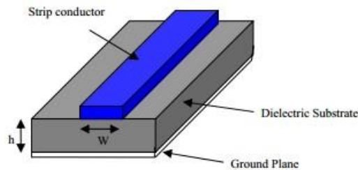
Gambar 2.2 Teknik Pencatuan Mikrostrip Line (Sumber : [4])
