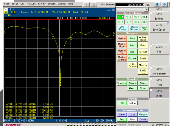
Gambar 3.2 Grafik Pengukuran Return Loss
