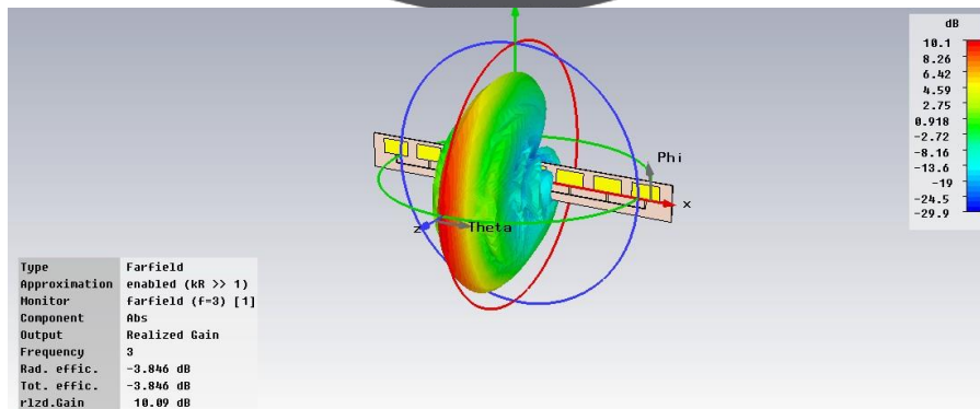
Gambar 2.6 Grafik Pola Radiasi dan Nilai Gain
