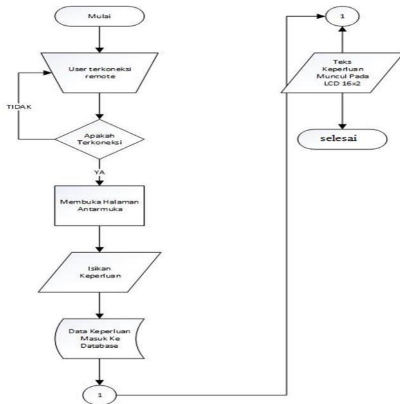
Gambar 3.4 Diagram Alir
