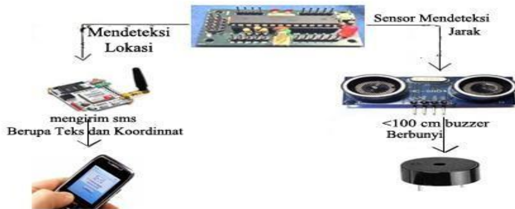
Gambar Blok Diagram Alat
