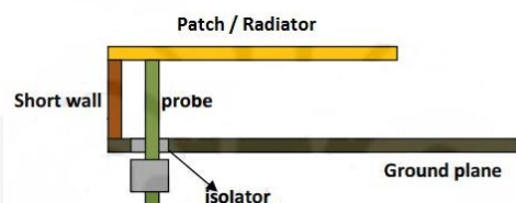
Gambar 1. Struktur antenna PIFA [5]
