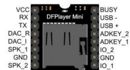
Gambar 2.2. Pin-pin pada Modul DFPlayer Mini
