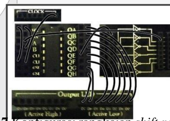
Gambar 7 Konfigurasi rangkaian shift register pada digital trainer
