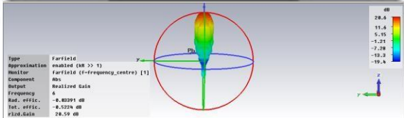
Gambar 3.12 Gain Hasil Optimasi Simulasi
