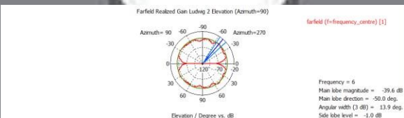
Gambar 3.15 Pola Radiasi Elevasi Hasil Optimasi Simulasi
