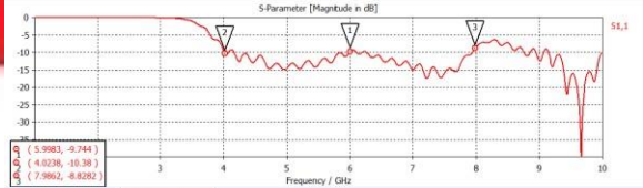
Gambar 3.10 Return Loss Hasil Optimasi Simulasi
