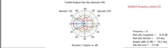
Gambar 3.14 Pola Radiasi Azimuth Hasil Optimasi Simulasi
