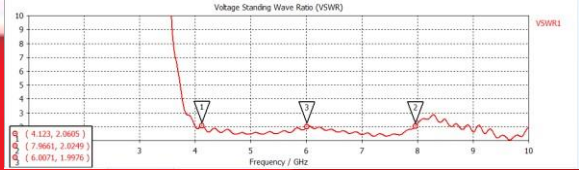
Gambar 3.9 VSWR Hasil Optimasi Simulasi
