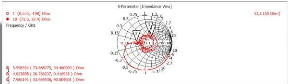
Simulasi Gambar 3.13 Polarisasi Hasil Optimasi Simulasi
