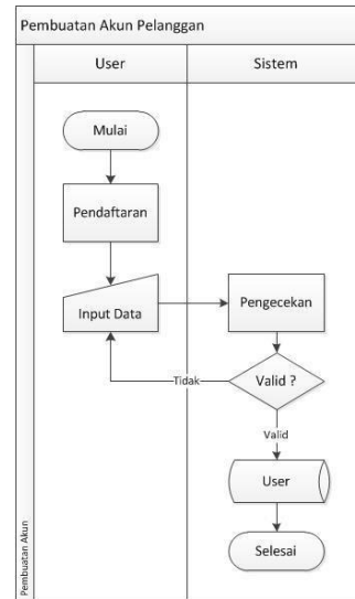
Gambar 3.5 Proses Pembuatan Akun
