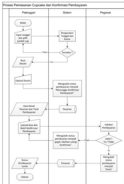
Gambar 3.7 Proses Pemesanan Cupcake dan Konfirmasi Pembayaran
