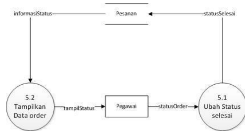
Gambar 3.18 Proses Perubahan Status Selesai
