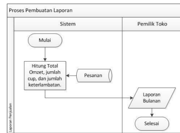
Gambar 3.10 Proses Pembuatan Laporan
