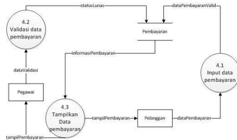
Gambar 3.17 Proses Konfirmasi Pembayaran
