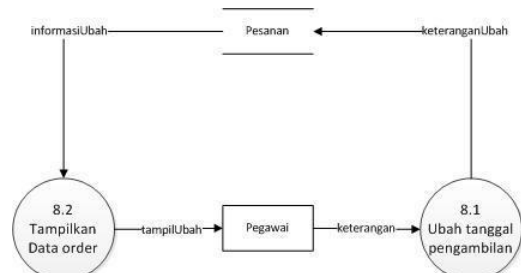
Gambar 3.19 Proses Perubahan Tanggal Pengambilan
