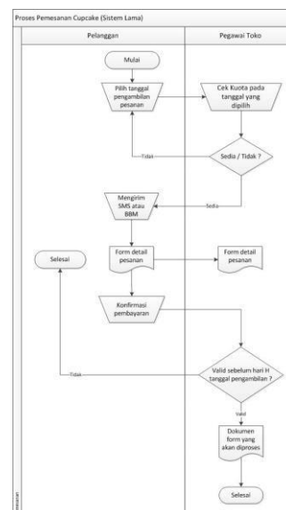
Gambar 3.1 Proses Pemesanan Cupcake (Sistem Lama)
