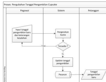
Gambar 3.11 Proses Pengubahan Tanggal Pengambilan
