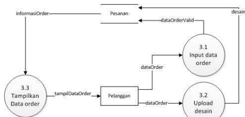
Gambar 3.16 Proses Pemesanan Cupcake
