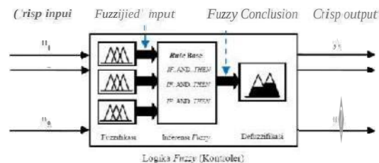
Gambar 2.1 Struktur Dasar Sistem Inferensi Fuzzy [7]
