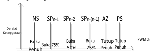
Gambar 2.3 Fungsi keanggotaan output
