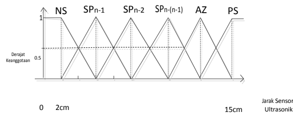
Gambar 2.2 Fungsi keanggotaan jarak sensor ultrasonik
